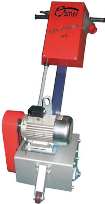
Décapeuse électrique MB 2000
