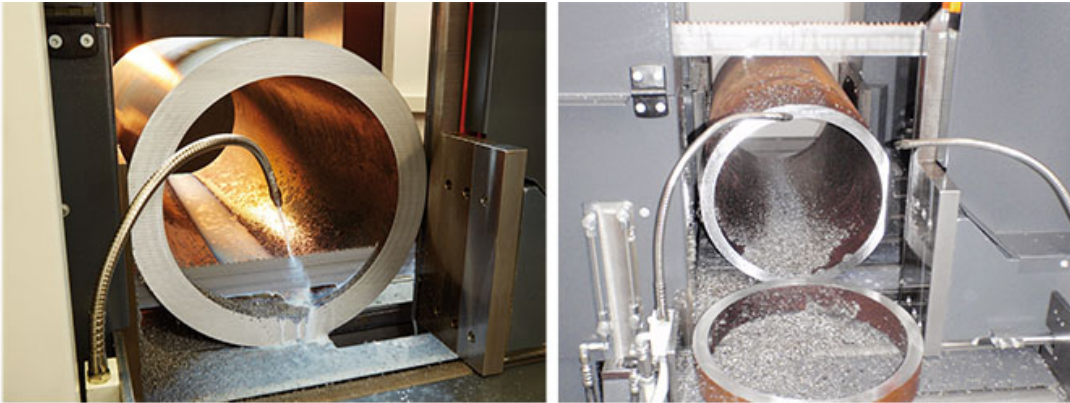
Le sciage du bas vers le haut de la KASTOwin tube A 5.0., une spécificité de ce modèle, procure un excellent état de surface de la pièce coupée.
