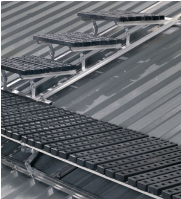
Le chemin de circulation pour toitures et terrasses
